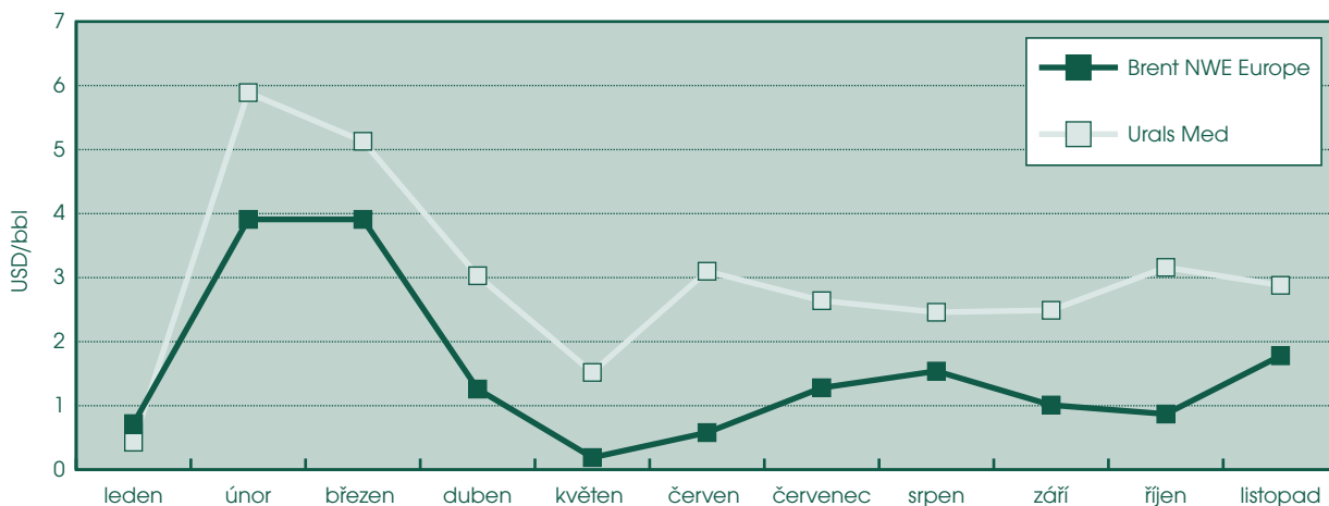
Graf 4: Rafinérské marže v roce 2003 – krak
