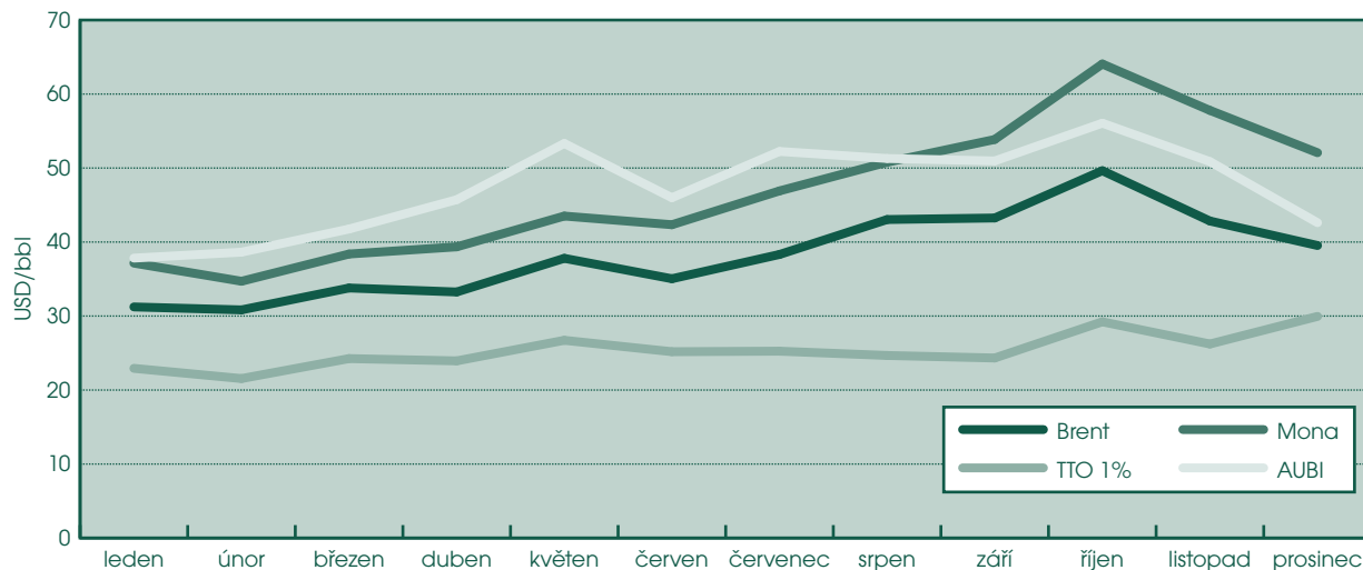
Graf 2: Ceny ropy a produktů v roce 2004 FOB Rotterdam Barges
